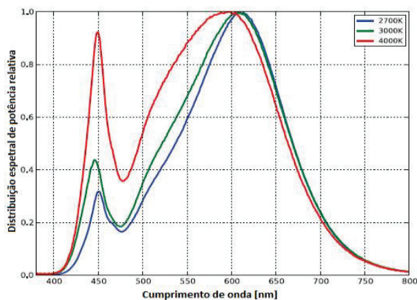
Figura 15 – Espectro do LED para as Temperatura de Cor 2.700 K, 3.000 K e 4.000 K[24]
